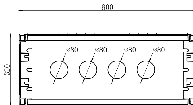
去门正视
